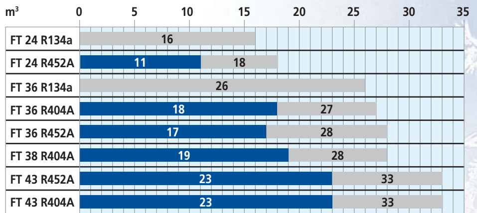
Frigo Top 24, 36, 38 ja 43 -laitteet rahtitilan koon mukaan @ 30°C
