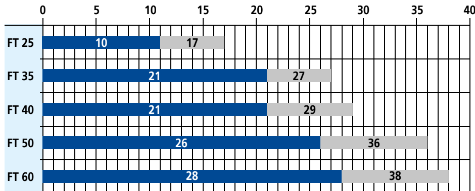
Frigo Top 25, 35, 40, 50 ja 60 -laitteet ajoneuvon koon mukaan @ 30°C ■ -20°C ■ 0°C
